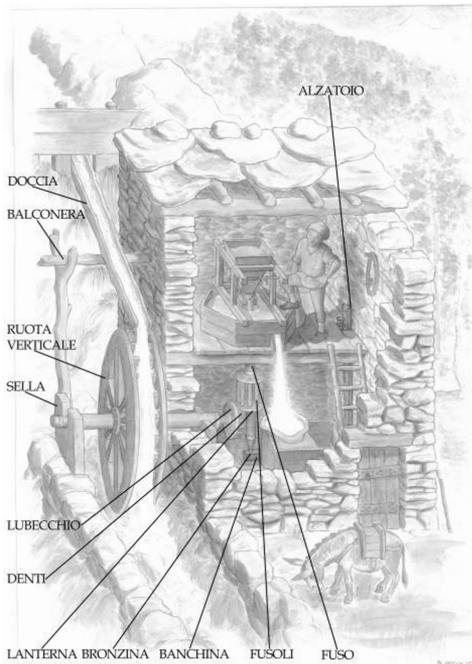
TAVOLA 2) Mulino a ruota verticale (Illustrazione di B. Orsello).
